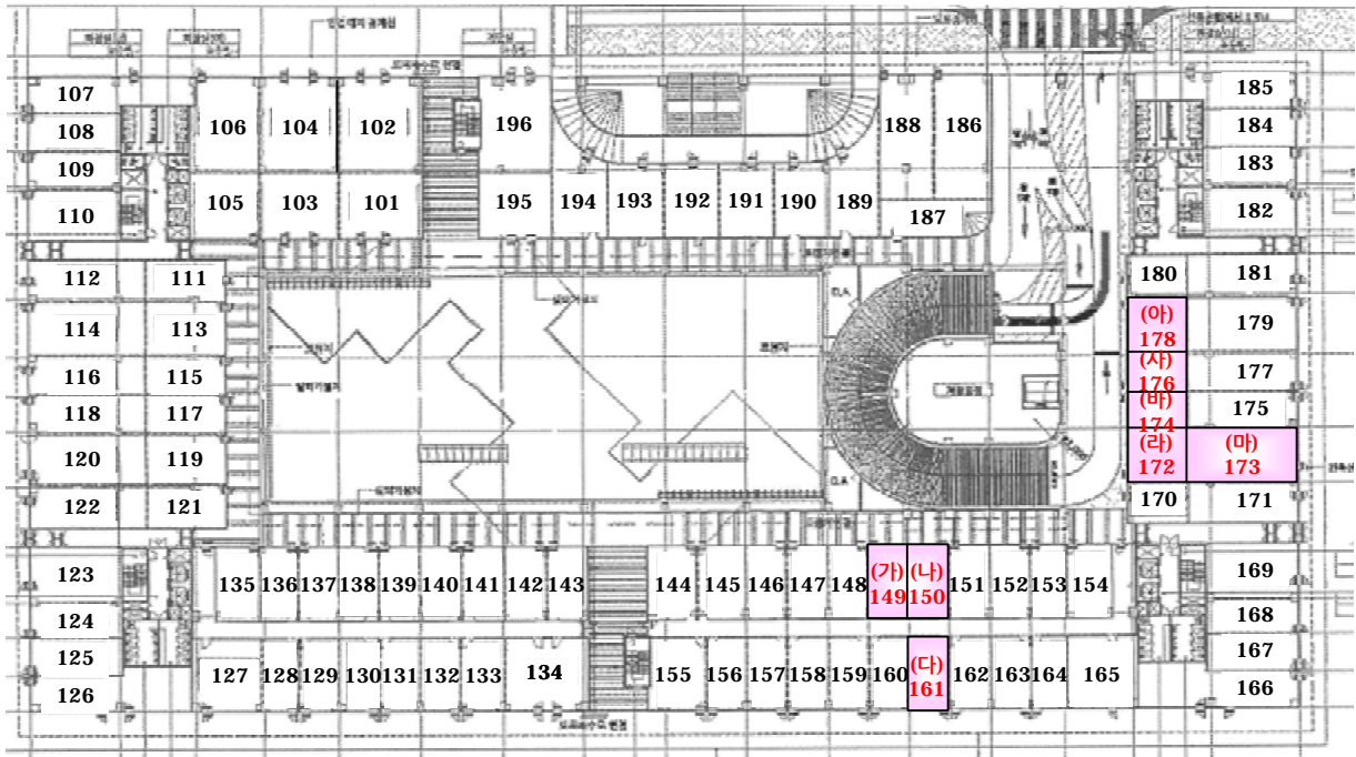
[ 제1층 호별배치도 및 제149호 외 내부구조도 ]
